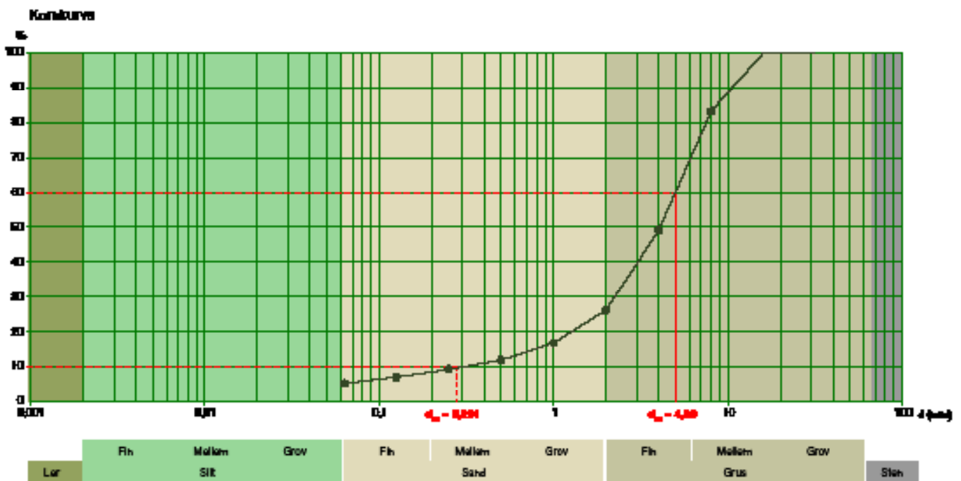
Eksempel på en kornkurve. Kurven viser et velgraderet materiale.
