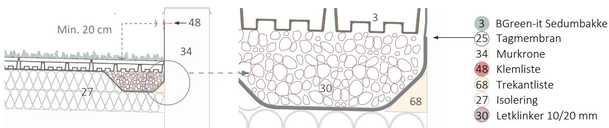
BGreen_it_60_Sedumbakker_Murkrone med lukket kasserende
