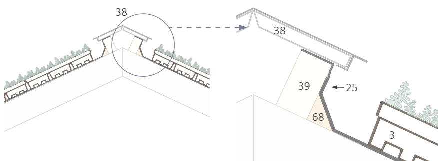
BGreen_it_60_Sedumbakker_Rygningsudluftning oplodset
