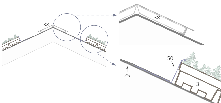
BGreen_it_60_Sedumbakker_Rygningsudluftning
