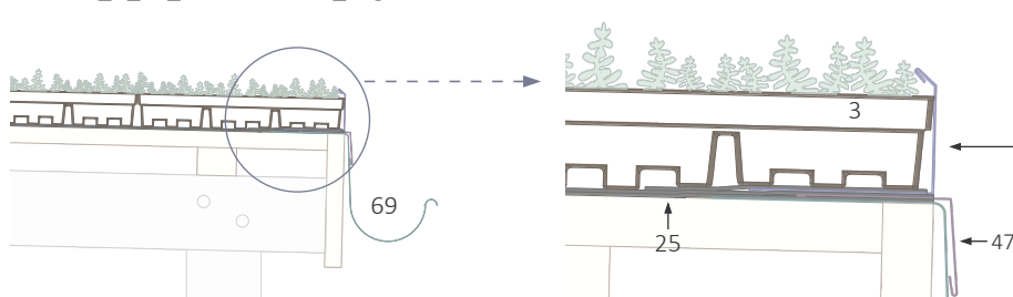
BGreen_it_60_Sedumbakker_Tagfod 1,4 - 10°
