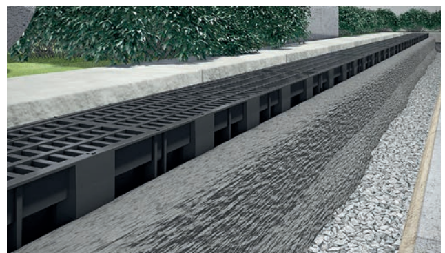
Understøt med beton
