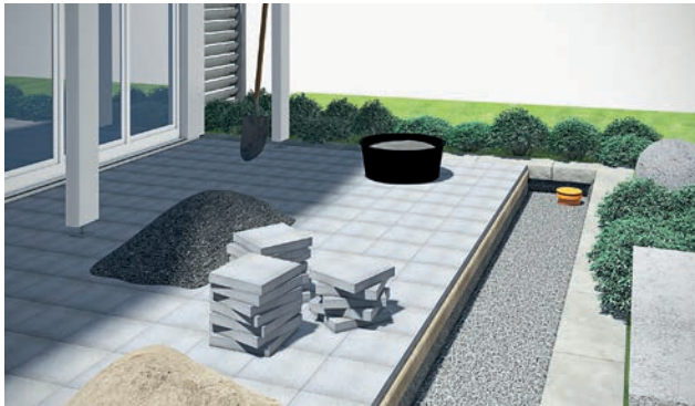
Udgravning med frostresistent underlag til ilægning af afvandringsrender
